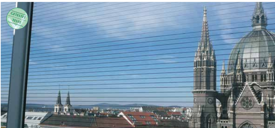
Vodorovné černé čáry tloušťky 2 mm s roztečí 28 mm vykazovaly v průřetovém tunelu navzdory všem očekáváním velmi dobré výsledky. Tam, kde je důležité zajistit co nejlepší viditelnost, např. před světlým pozadím, jsou přijatelným řešením. Doporučovali bychom však tloušťku čar alespoň 3 mm.
